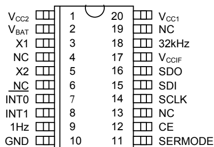
DS1306 20-Pin TSSOP (4.4mm)
